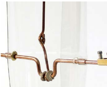
Abb. 202 | Schubstange mit Pleuel, geführt mit Kartonunterlagsscheiben
