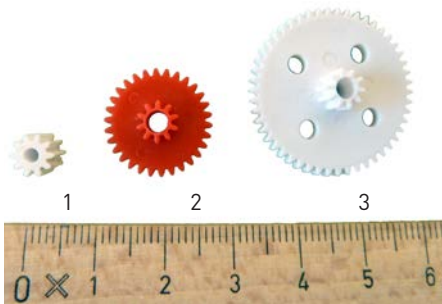
Abb. 213 | Doppelzahnrad Modul 0,5
